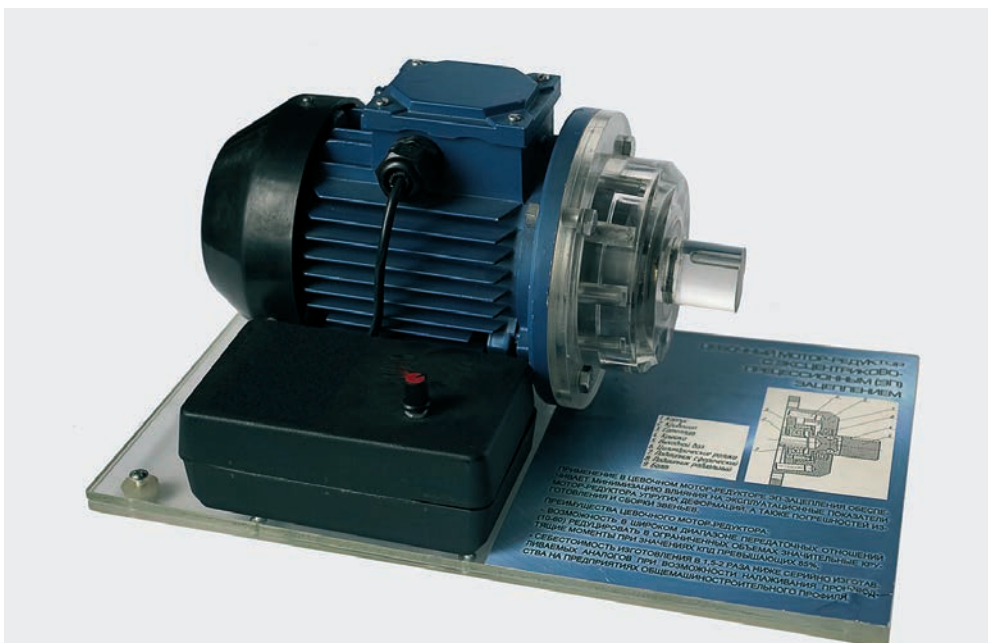
Прецессионный мотор-редуктор
