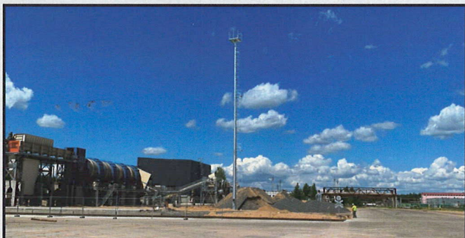
Мачта с площадкой и лестницами, 30 м, компания «Кроноспан», г. Сморгонь
