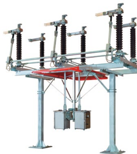
Разъединитель горизонтально-поворотного типа РГ(Н)-СВЭЛ-110
